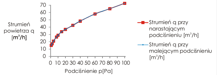
Wykres 1. Zależność strumienia powietrza q [m 3 /h] przepływającego przez nawiewnik VT 101 od panującego podciśnienia p [Pa]
