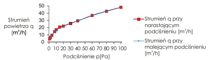
Wykres 2. Zależność strumienia powietrza q [m 3 /h] przepływającego przez nawiewnik VT 201 od panującego podciśnienia p [Pa]
