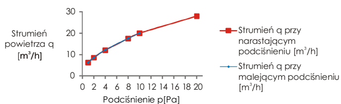
Wykres 4. Zależność strumienia powietrza q [m 3 /h] przepływającego przez nawiewnik VT 601 od panującego podciśnienia p [Pa]
